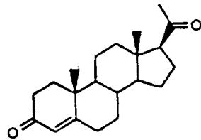
Progesterone
